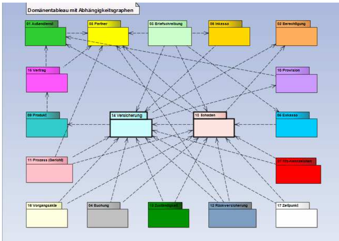
Abbildung Domänentableau des ASSKURA-Modells
